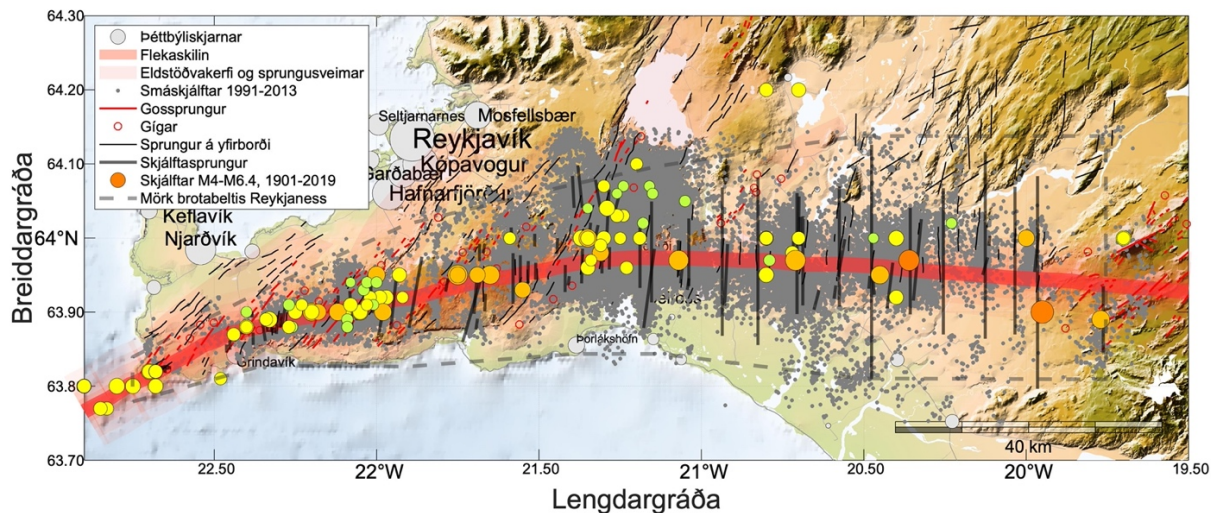
Mynd 3. Afstaða höfuðborgarsvæðisins til brotabeltis Suðurlands og Reykjanes, flekaskilanna, og áætluðum mörkum brotabeltisins (sjá myndatexta við Mynd 2).
