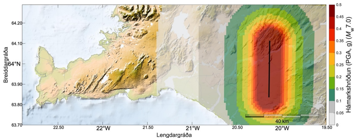
Mynd 7 (framhald). Reiknuð hámarkshröðun yfirborðs jarðar í sviðsmyndum jarðskjálfta skv. hámarksstærð skjálfta eftir staðsetningu frá vestri til austurs eftir brotabelti Suðurlands og Reykjanes (Tafla 1). Gildi og afstaða hámarkshröðunar byggir á meðaltali dvínunarlíkinganna á Mynd 6 og ráðandi NS-stefnu þvergengja hverra miðjur liggja á flekaskilunum. Staðsetning sviðsmyndar hvers svæðis er slemmbivalin innan marka brotabeltisins.
