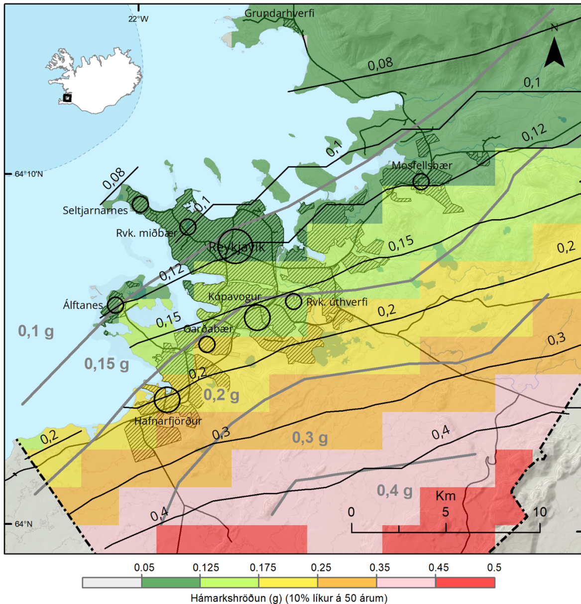
Mynd 21. Grófur samanburður á uppfærðu skjálftavárlíkindakorti á höfuðborgarsvæðinu (litir og svartar jafngildislínur) og núgildandi skjálftavárlíkinda skv. Þjóðarskjali Íslands fyrir Eurocode 8 (gráar línur sem skilja að svæði með mismunandi hámarks hröðun). Kortið sýnir hámarks hröðun á yfirborði jarðar sem er með 10% líkur á umframgildi á 50 ára tímabili.
