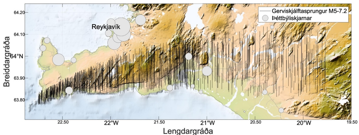
Mynd 8. Dæmi um hermda gerviskjálftaskrá fyrir 3000 ára tímabil með slembiúrtökum staðsetninga norður-suður þvergingja á brotabelti Suðurlands og Reykjaness skv. hinu nýja jarðskjálftalíkani. Staðsetningar og umfang gerviskjálfta á stærðarbilinu M_w 5-7,2 eru sýndar með svörtum heildregnum línum.
