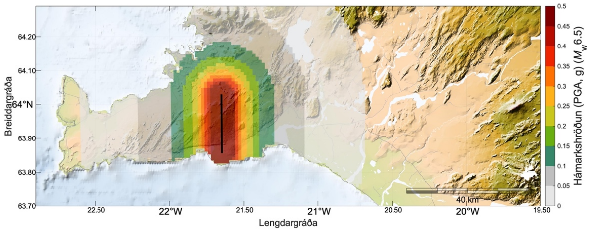
Mynd 7. Reiknuð hámarksþröðun yfirborðs jarðar í sviðsmyndum jarðskjálfta skv. hámarksstærð skjálfta eftir staðsetningu frá vestri til austurs eftir brotabelti Suðurlands og Reykjaness (Tafla 1). Gildi og afstaða hámarksþröðunar byggir á meðaltali dvinunarlíkinganna á Mynd 6 og ráðandi NS-stefnu þvergengja hverra miðjur liggja á flekaskilunum. Staðsetning sviðsmyndar hvers svæðis er slembivalin innan marka brotabeltisins.
